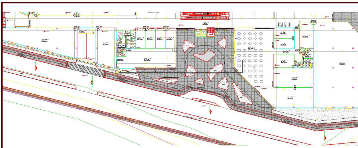
Figura 6 - Projeto de acesso do empreendimento.
